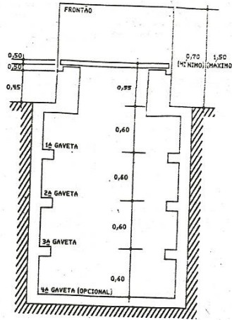
CORTE AA
