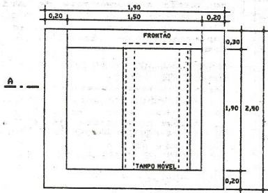
PLANTA TÉRREO
