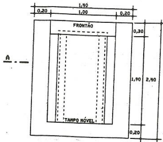
PLANTA TÉRREO
