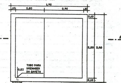
PLANTA SUBSOLO
