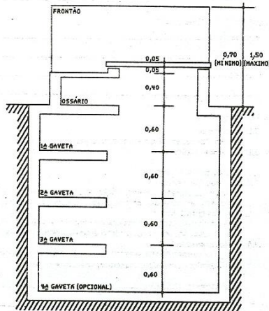
CORTE AA
