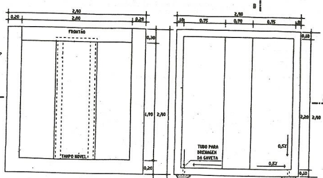
PLANTA TÉRREO
