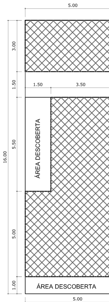
PLANTA SUPERIOR
