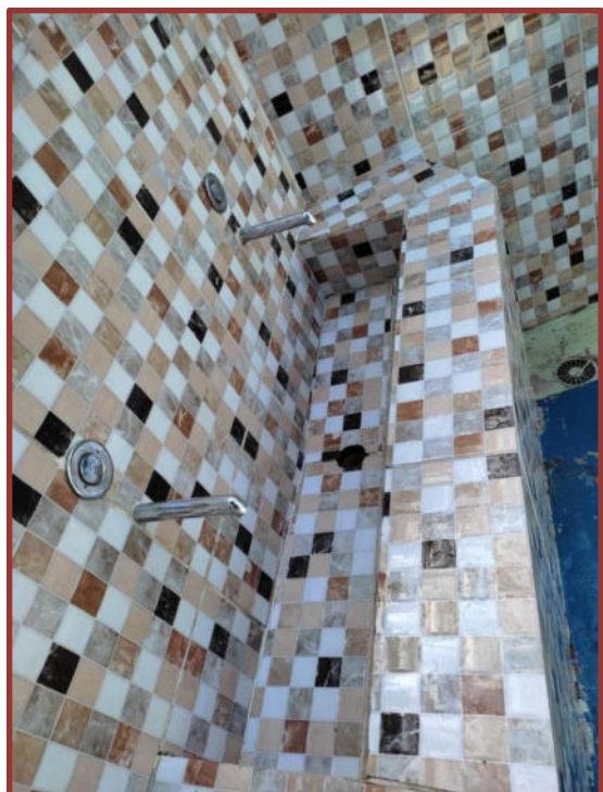
Figura 17 – Instalação de torneira de fechamento automático tipo parede – antivandalismo em unidade escolar
