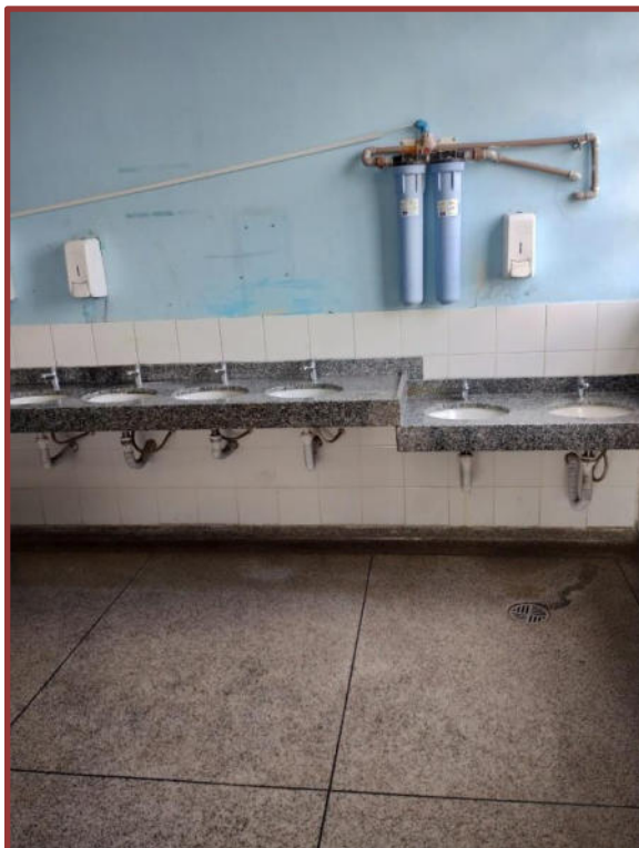
Figura 15 – Instalação de torneiras de fechamento automático tipo mesa em unidade escolar
