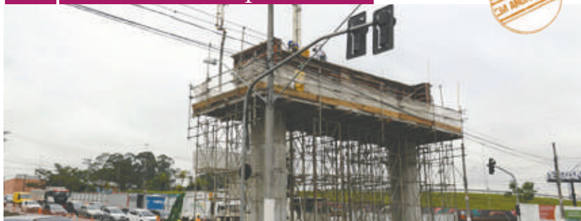
DUPLICAÇÃO DA RUA JOSÉ ODORIZZI FAZENDO LIGAÇÃO COM A SAMUEL AIZEMBERG E IMIGRANTES. (CORREDOR LESTE-OESTE)
